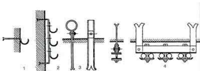
Сл. 39. Кабловска обујмица: 1 – једнострука отворена, 2 – вишеструка отворена, 3 – једнострука затворена, 4 – вишеструка полуотворена
