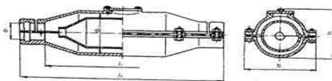
Сл. 37. Права оклопна спојница са унутрашњом оловном, за радни напон до 1 кV: 1 – цртеж спојнице у две пројекције; 2 – спојница са прибором за монтажу (везни жица, уље за уземљење), изолациона трака, импрегнирани папир, азбестна трака, јутана трака, паста за демљење, стеари и маса за валцање, унутрашње и спољне заштитне спојнице
