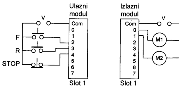
Šema veze
