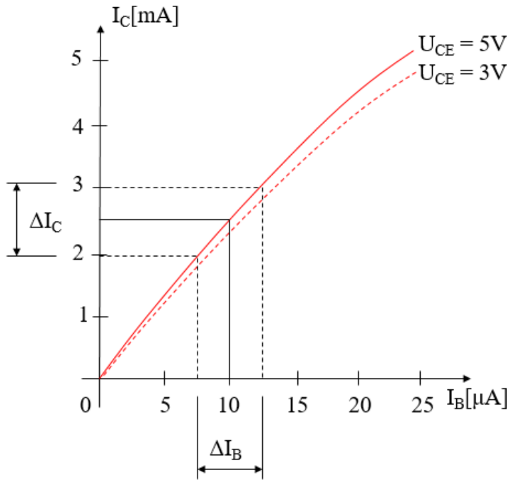
Слика 3 Преносне карактеристике транзистора
